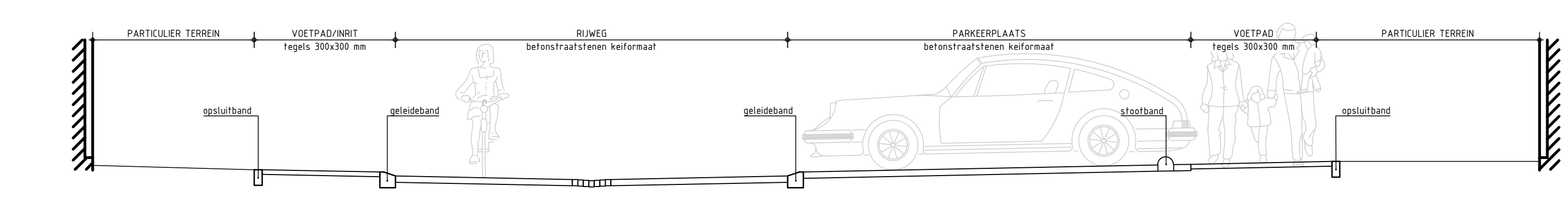
DOORSNEDE RUITENVEEN SCHAAL 1:50
